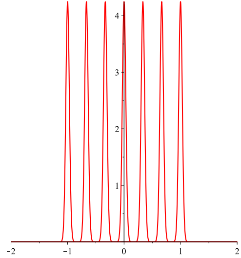
Рис. 4: счетная система векторов \phi_{n,\epsilon}(x) , для \epsilon = 1/32 .
